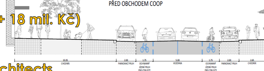
C - C' - ULIČNÍ PROFIL UL. VÍTA NEJEDLÉHO PŘED DOMEM Č.P. 920/921
