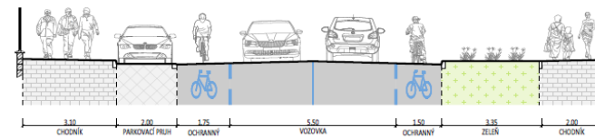
B - B' - ULIČNÍ PROFIL UL. VÍTA NEJEDLÉHO PŘED OBCHODEM COOP
